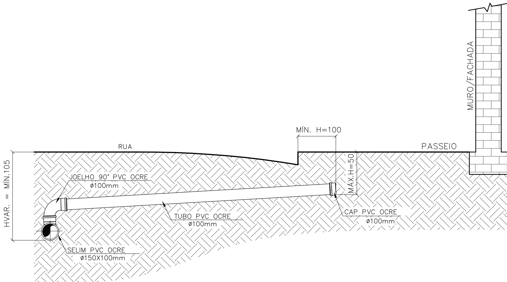
DETALHE TÍPICO RAMAL DE LIGAÇÃO ESC. 1:20
