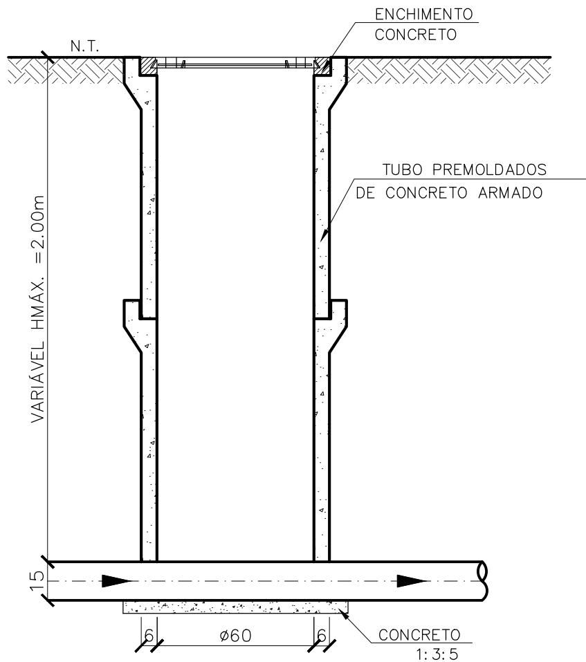
POÇO DE VISITA < 2,00m TUBO CONCRETO ARMADO ESC. 1:20
