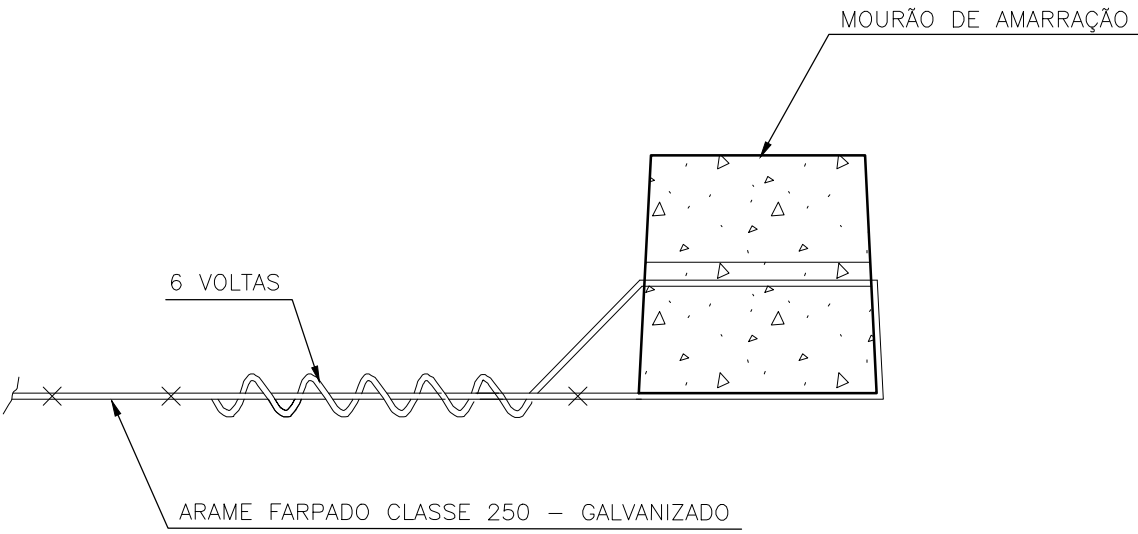
SEÇÃO B-B MOURÃO DE CONCRETO ARMADO ESC. 1:5
