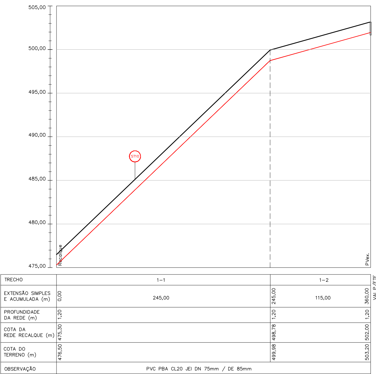
PERFIL LONGITUDINAL REDE RECALQUE DA ELEVATÓRIA ESC. HORIZONTAL 1:2.500 ESC. VERTICAL 1:250
