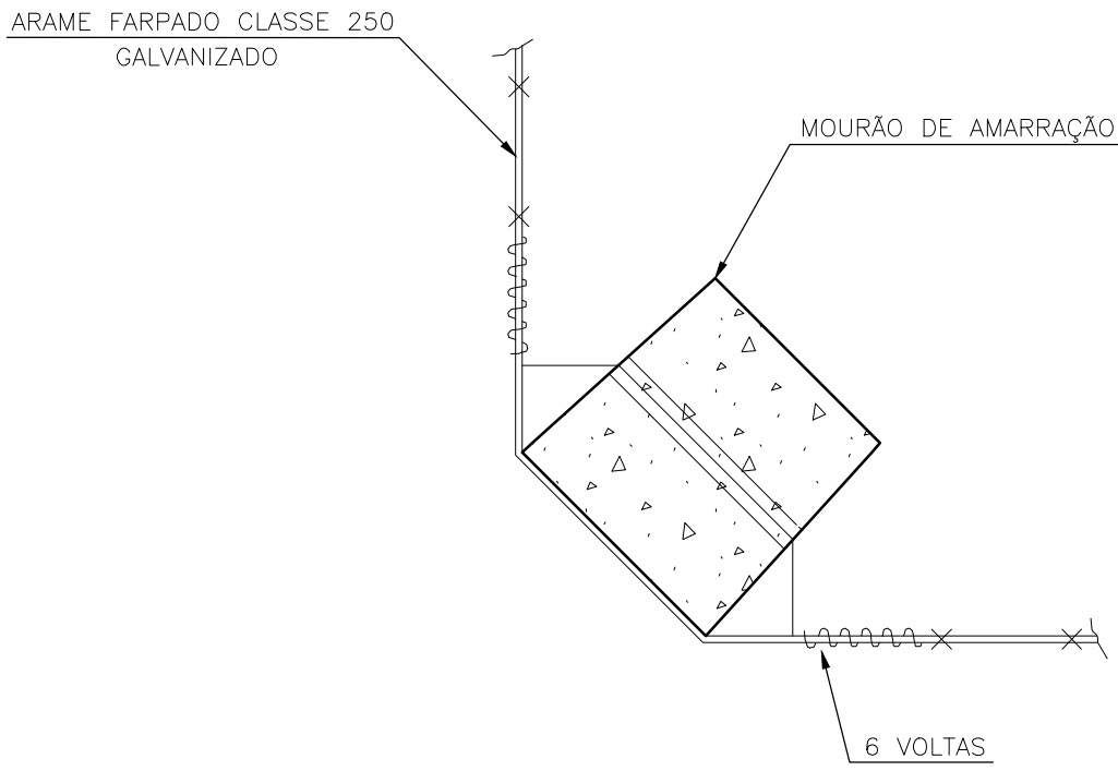
SEÇÃO A-A MOURÃO DE CONCRETO ARMADO ESC. 1:5
