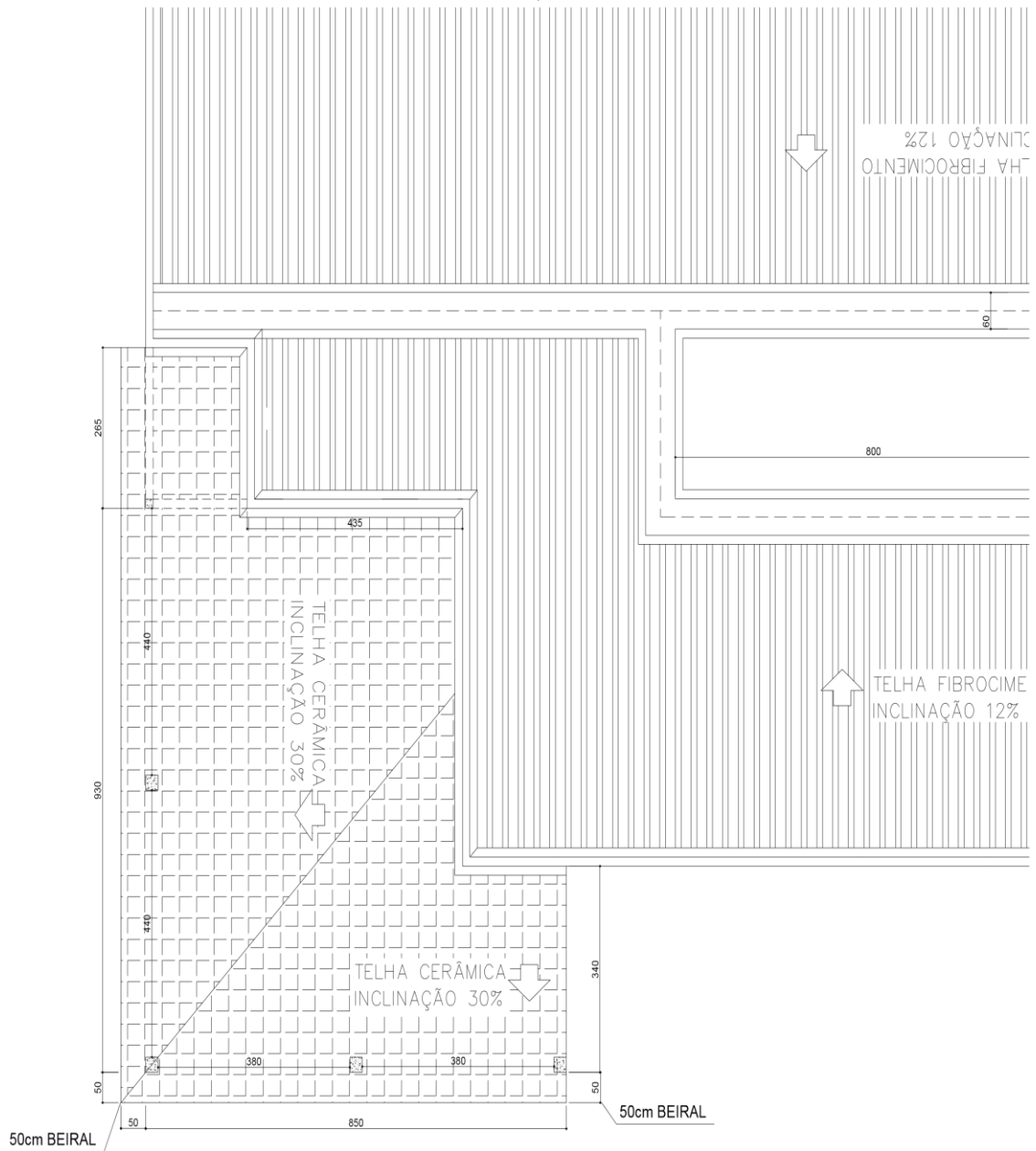
PLANTA PLANTA ESC 1:50
